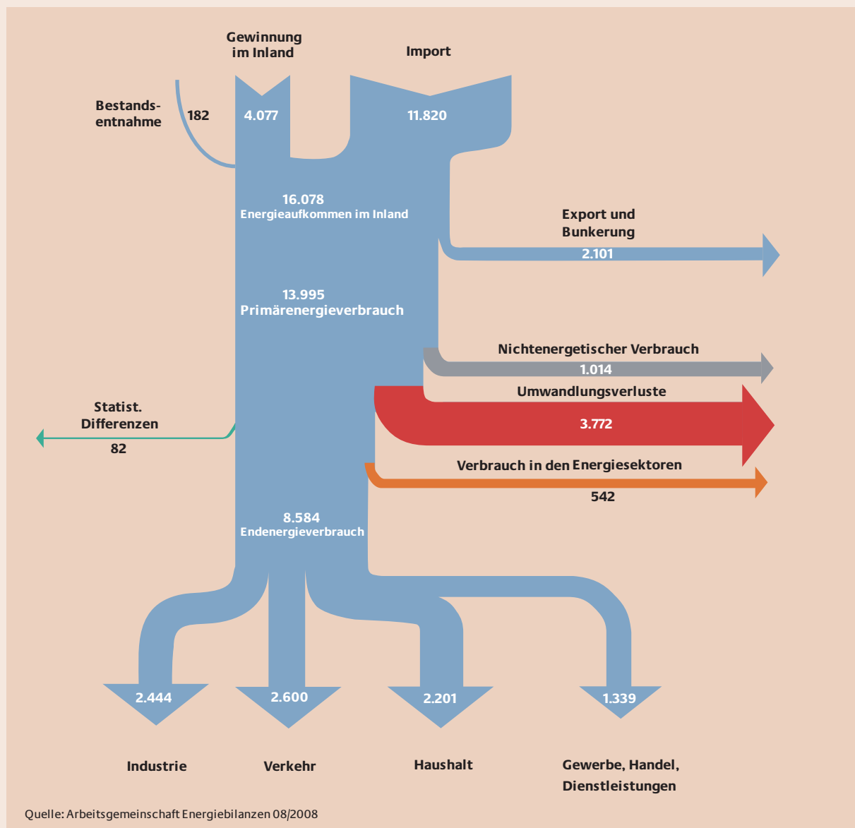
Schaubild 10: Energieflussbild 2007 Deutschland, in PJ
