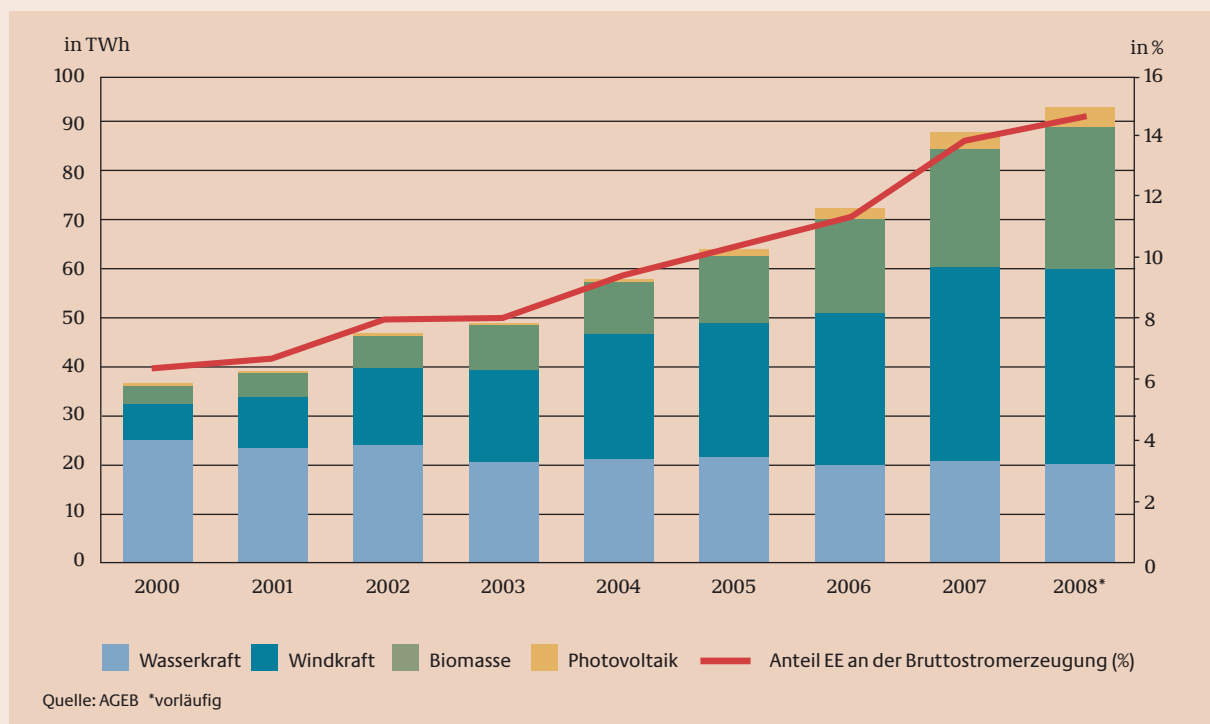
Schaubild 12: Bruttostromerzeugung aus erneuerbaren Energiequellen 2000 – 2008, in TWh
