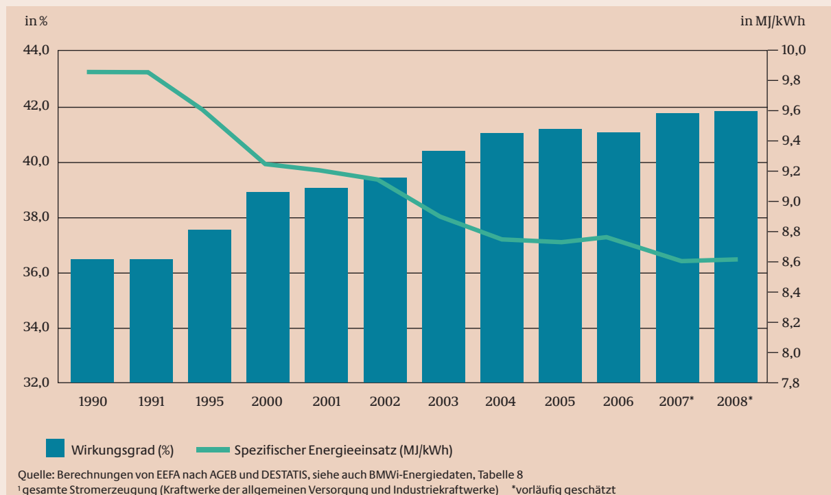
Schaubild 16: Wirkungsgrad und spezifischer Energieeinsatz der Stromerzeugung 1 in Deutschland 1990–2008, in % und MJ/kWh
