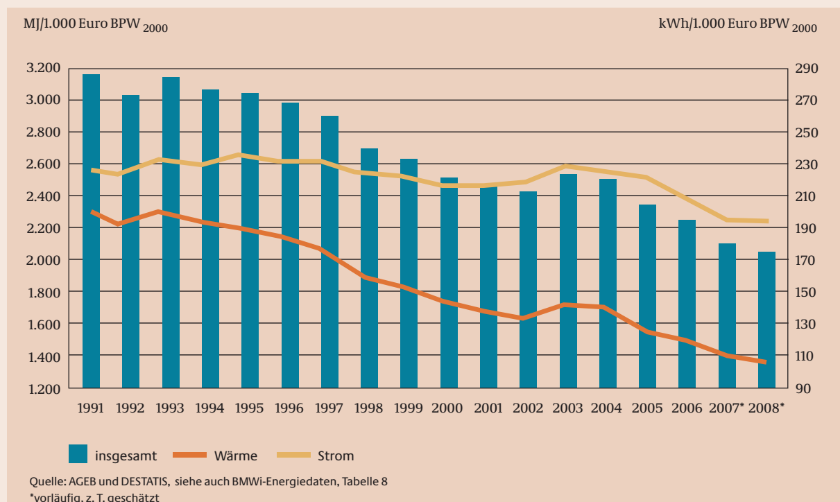
Schaubild 17: Entwicklung der Energieeffizienz der Industrie in Deutschland je Einheit Bruttoproduktionswert (BPW) in Preisen von 2000 1991–2008, MJ bzw. kWh/1.000 Euro BPW 2000
