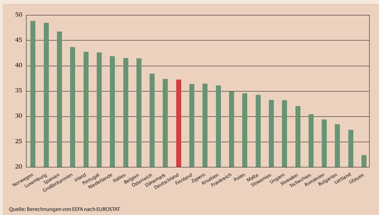
Schaubild 42: Wirkungsgrade konventioneller Wärmekraftwerke im europäischen Vergleich 2006, durchschnittliche Wirkungsgrade in %
