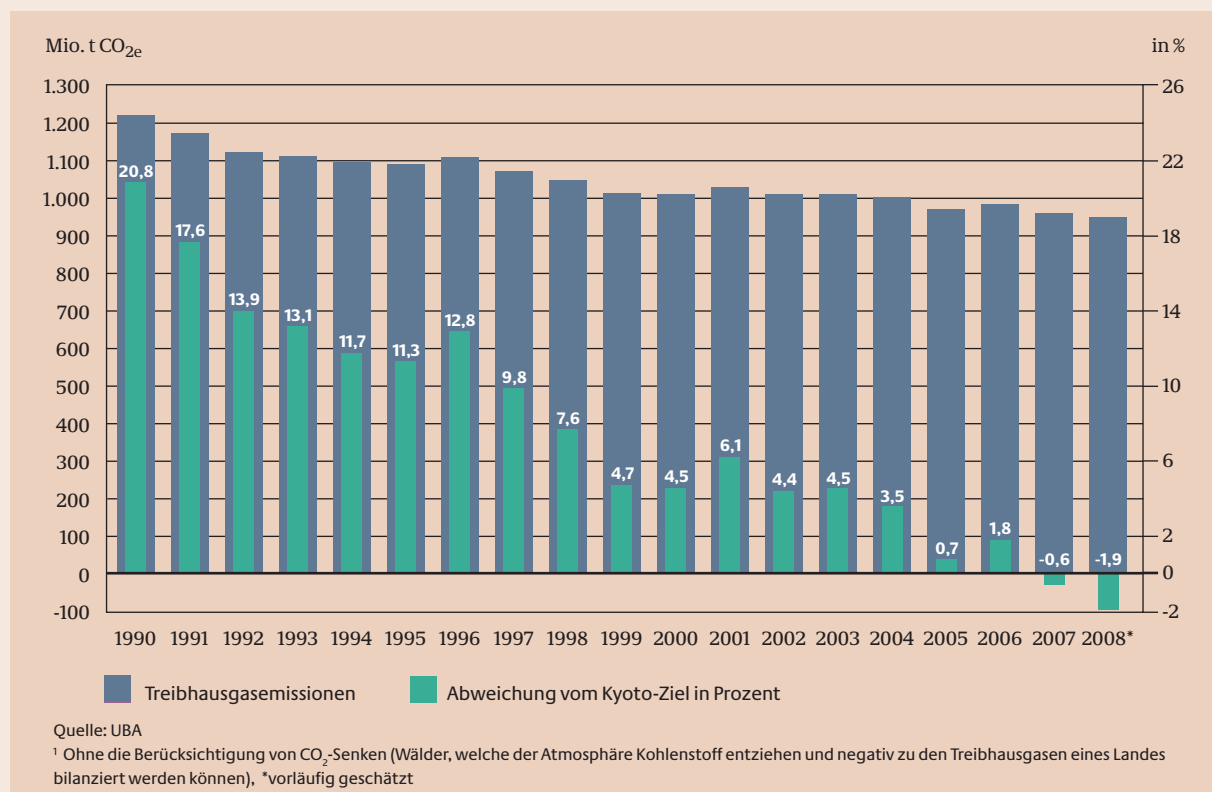
Schaubild 34: Entwicklung der Treibhausgasemissionen in Deutschland und deren Abweichung vom Kyoto-Minderungsziel 1 1990–2008, in Mio. t CO 2 -Äquivalente(CO 2e ) und %
