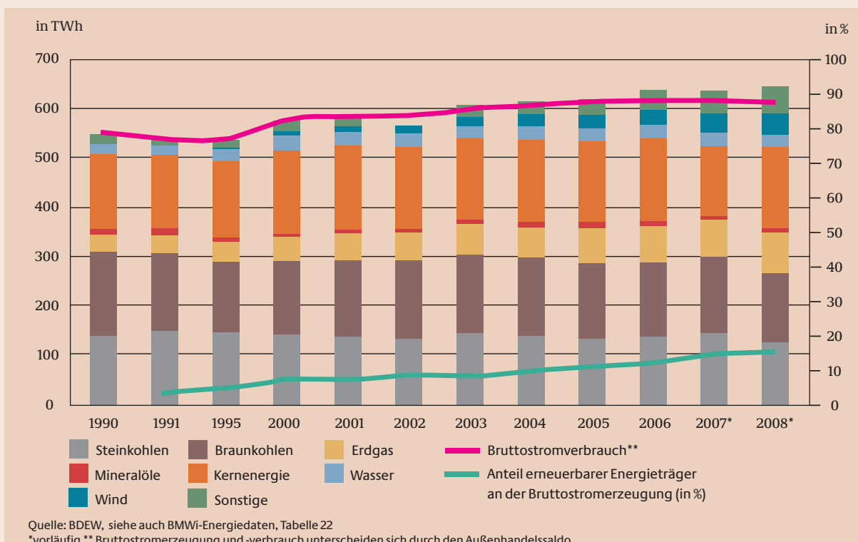
Schaubild 11: Bruttostromerzeugung aller Kraftwerke in Deutschland nach Energieträgern 1990–2008, in TWh und in %
